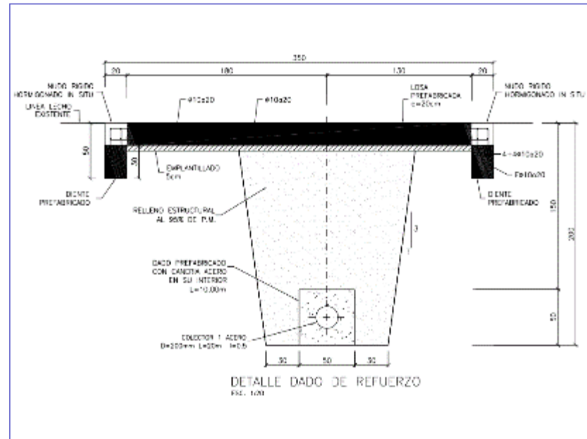
Losa protección en Canal Espejo
