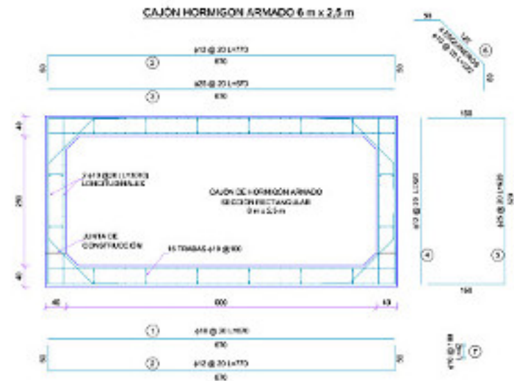
Sección Cajón H.A. Proyectoado.
