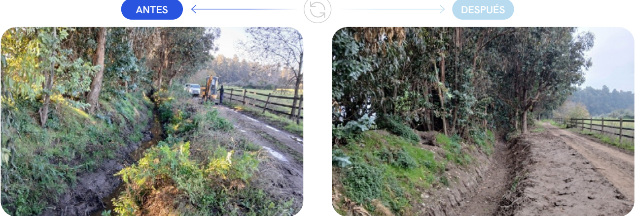
Canal Ochagavía, Derivado Délano, limpieza sector La Cruz, comuna Calera de Tango.
