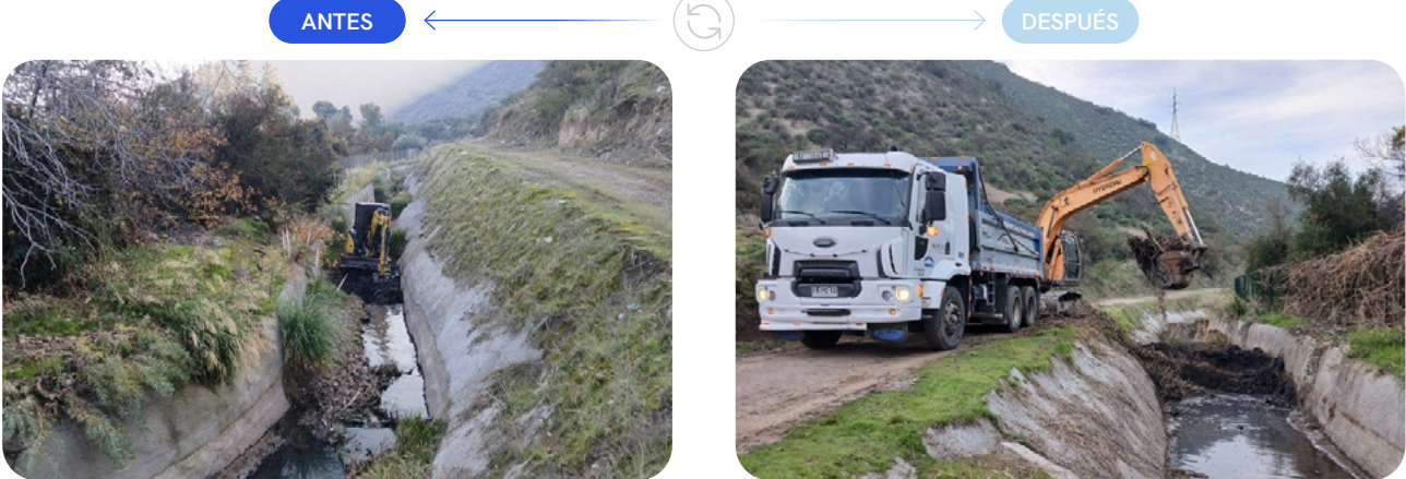
Canal Calera, limpieza sector Tanguito, comuna Calera de Tango.
