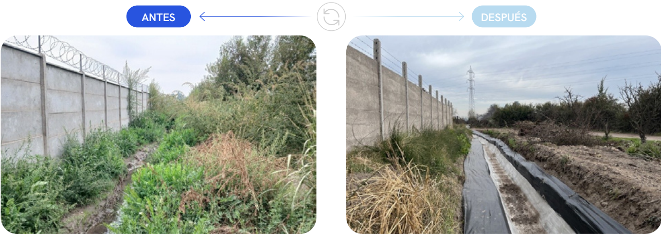
Revestimiento mediante Manta de hormigón Derivado San José de Tango, comuna Calera de Tango.
