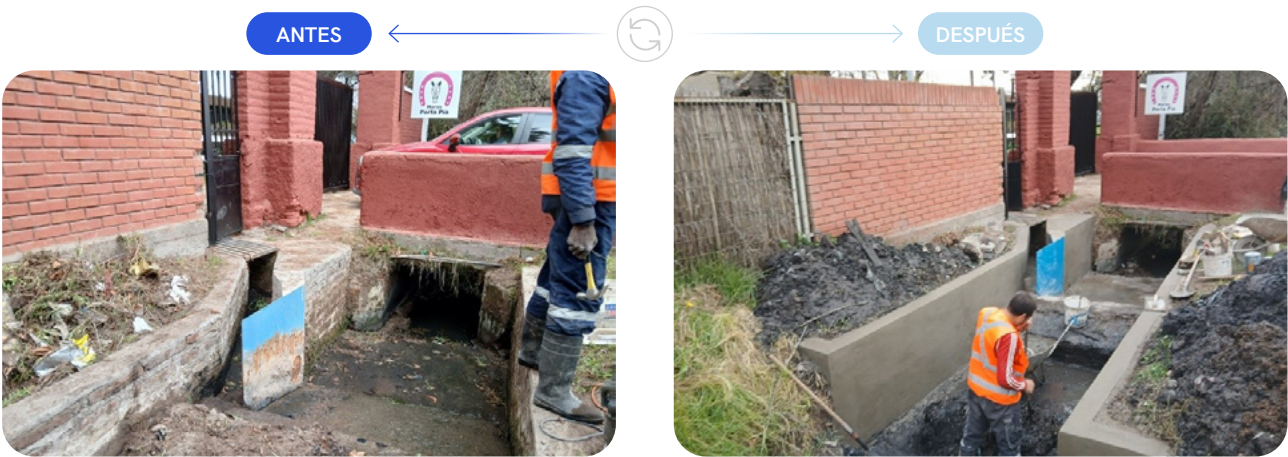
Reparación maro partidor M127 en canal Derivado San Javier, comuna Calera de Tango.
