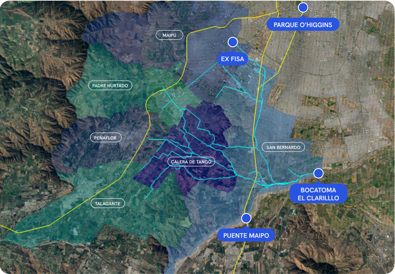
RED DE CANALES ASOCIACION CANALES DE MAIPO EN LA REGION METROPOLITANA
